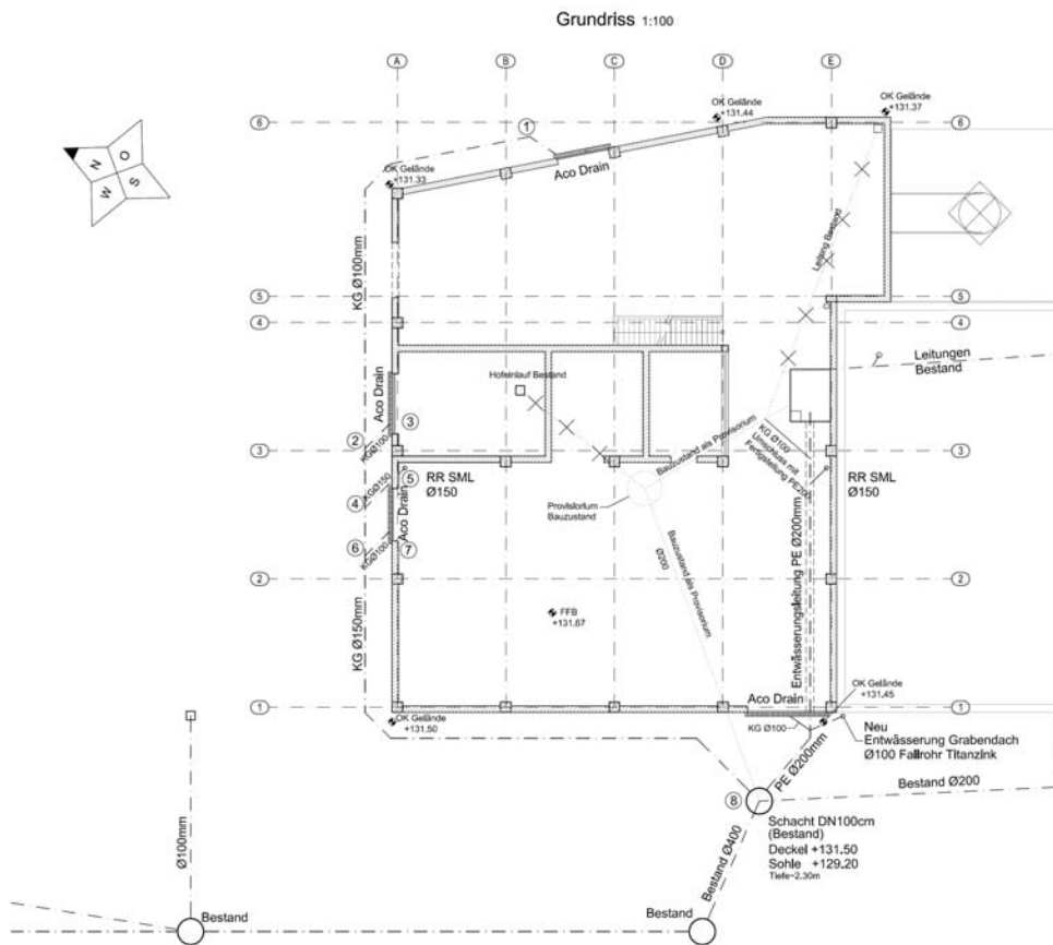
Grundriß Kraftwerksgebäude © rmd-consult
